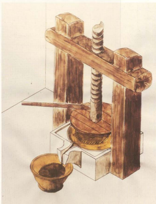
Restitution graphique du pressoir à vis de la parfumerie de Paestum (dessin Jean-Pierre Brun)
